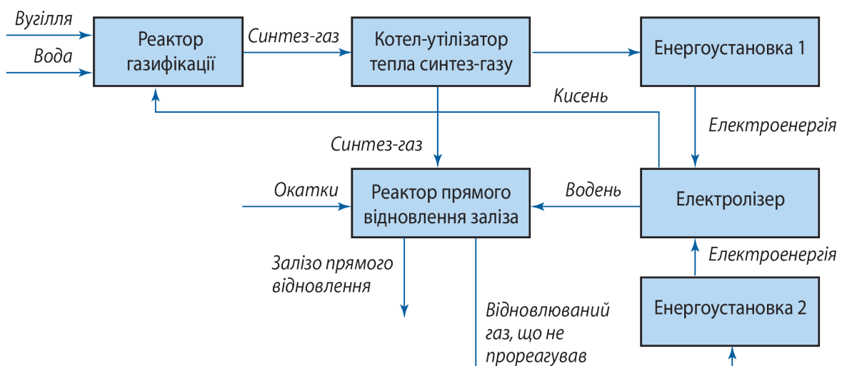
Рис. 4. Узагальнена схема запропонованої технології отримання заліза прямого відновлення
