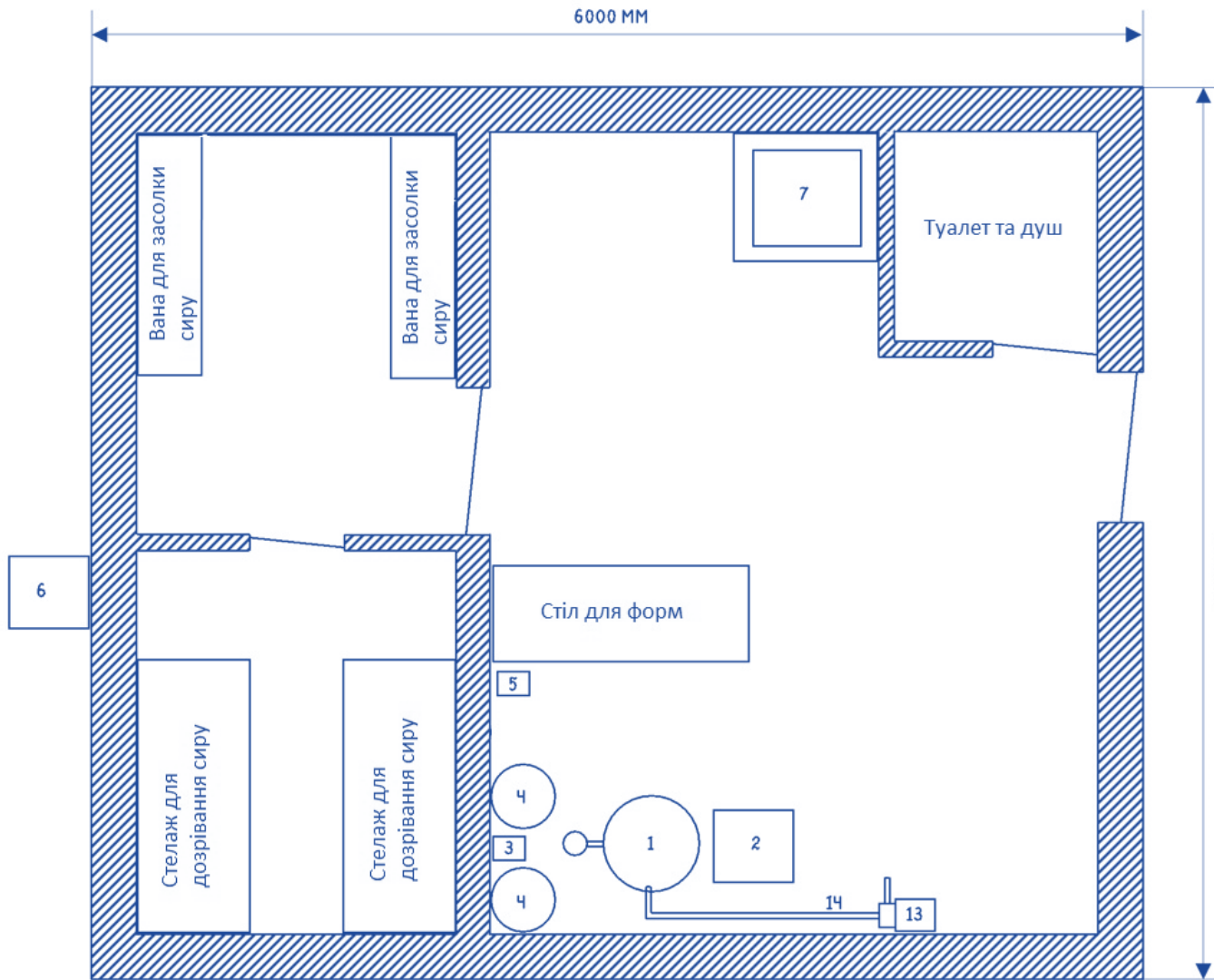
Рис. 1.2 План приміщення сироварні
